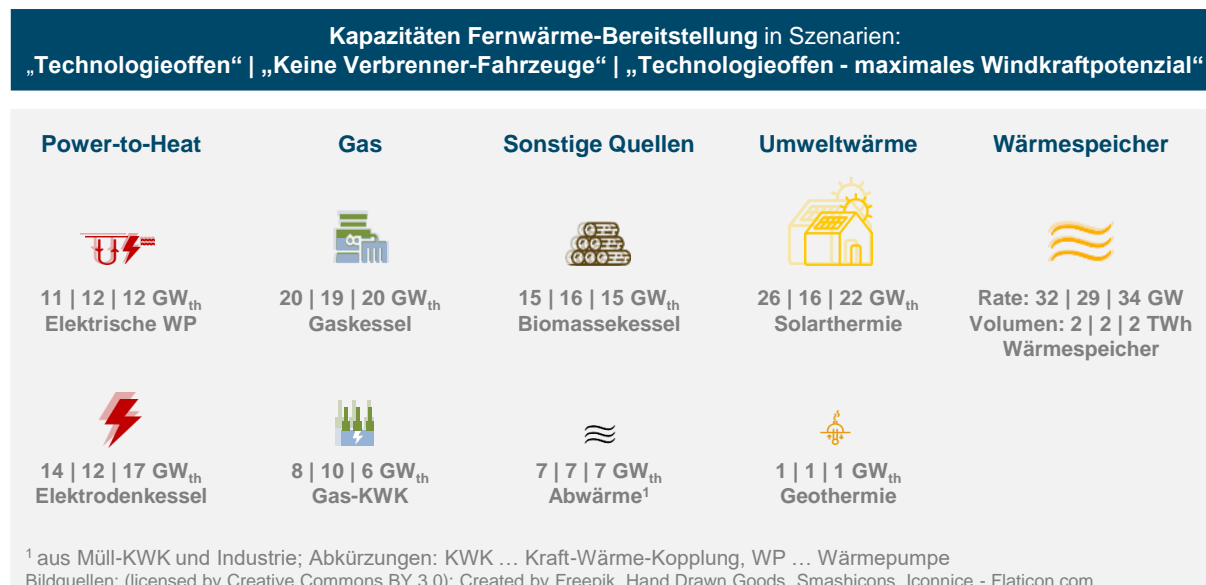
Abbildung 1-5: Technologiemitmix Fernwärme im optimierten Energiesystem in drei Szenarien
