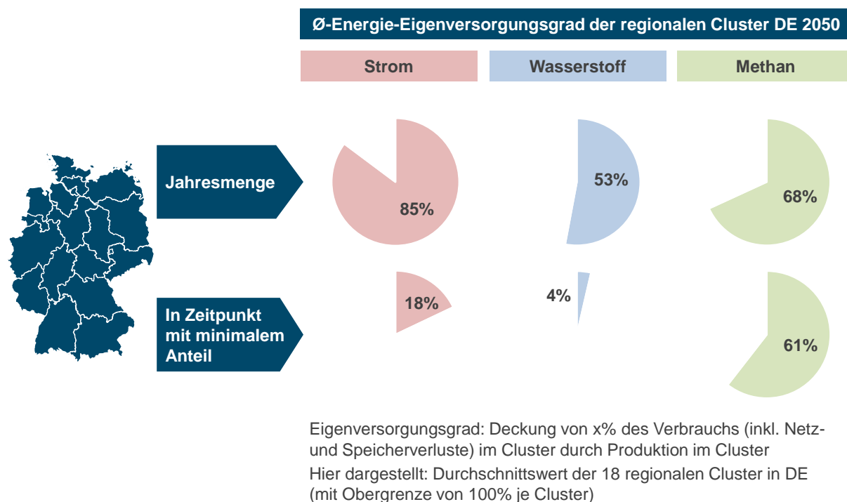
Abbildung 5-24: Durchschnittliche Energie-Eigenversorgungsgrade der Cluster im optimierten Energiesystem des Szenarios „Technologieoffen“
