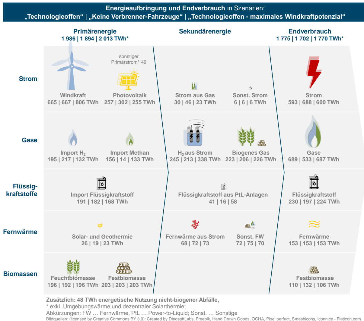
Abbildung 1-2: Überblick Energieaufbringung und Endverbrauch im optimierten Energiesystem in drei Szenarien – alle Angaben gerundet auf Zehnerstellen
